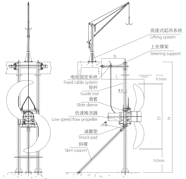
V 型安装
