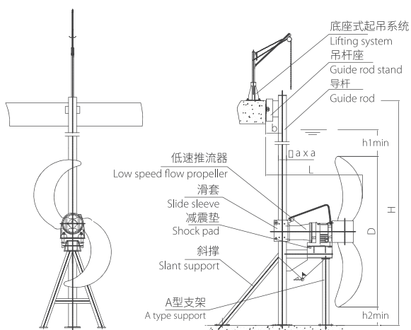
VI 型安装
