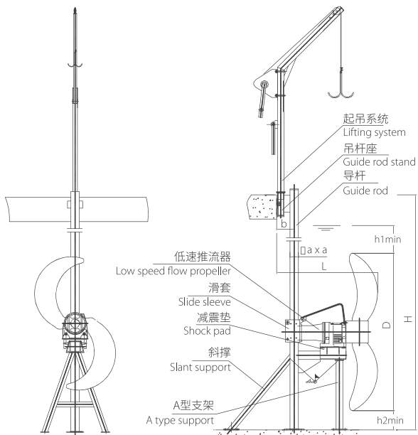
IV 型安装
